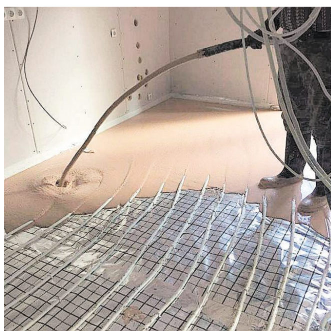
Spezieller Estrich beschleunigt die Installation und Inbetriebnahme einer Fußbodenheizung beträchtlich. Foto: Rapid-Floor Estrichtechnologie
